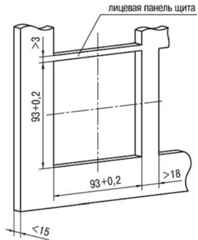
Рисунок А.2 – Прибор щитового крепления в корпусе типа Щ1
