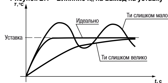
Рисунок Б.2 – Влияние T_i на выход на уставку
