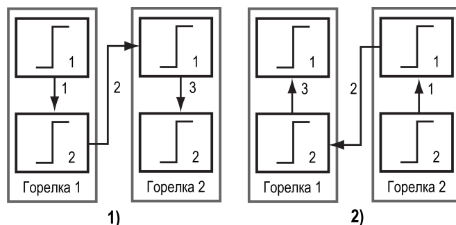
Рисунок 8.3 – Регулирование температуры по алгоритму «1212»: 1) включение, 2) выключение
