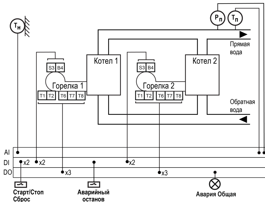
Рисунок 1.1 – Объект управления
