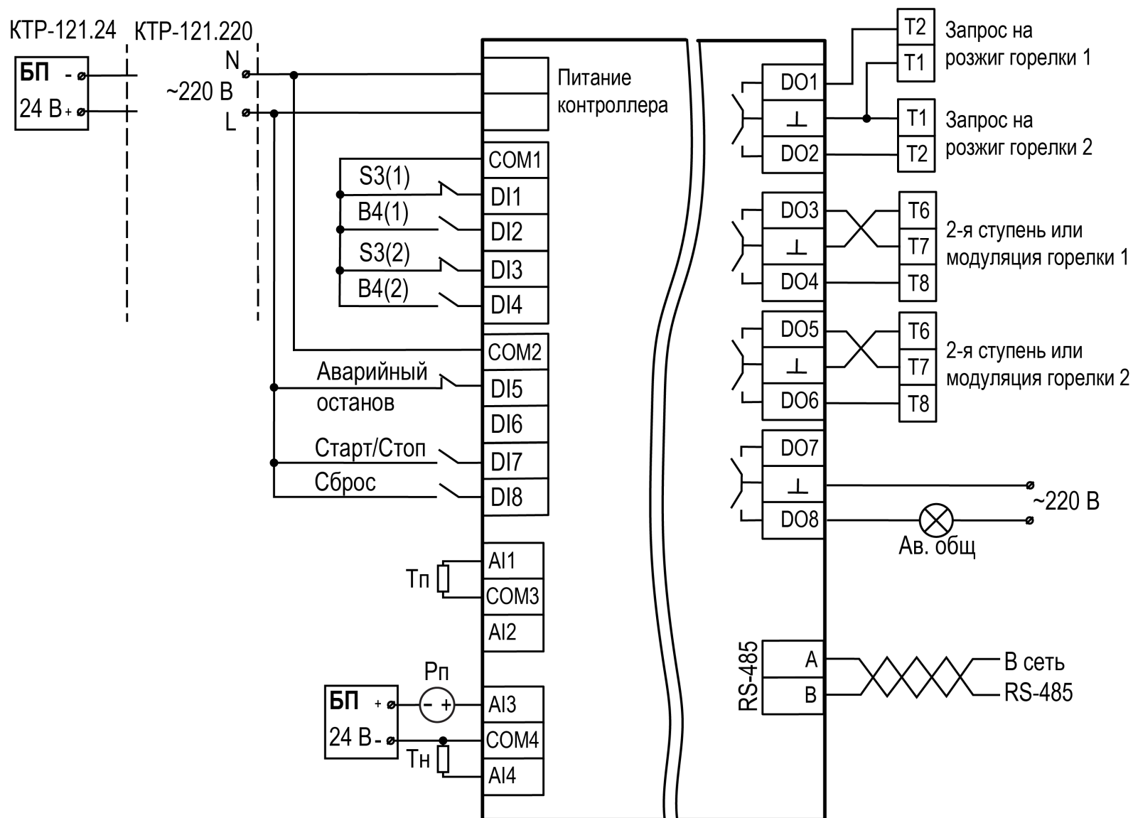
Рисунок 5.4 – Схема подключения
