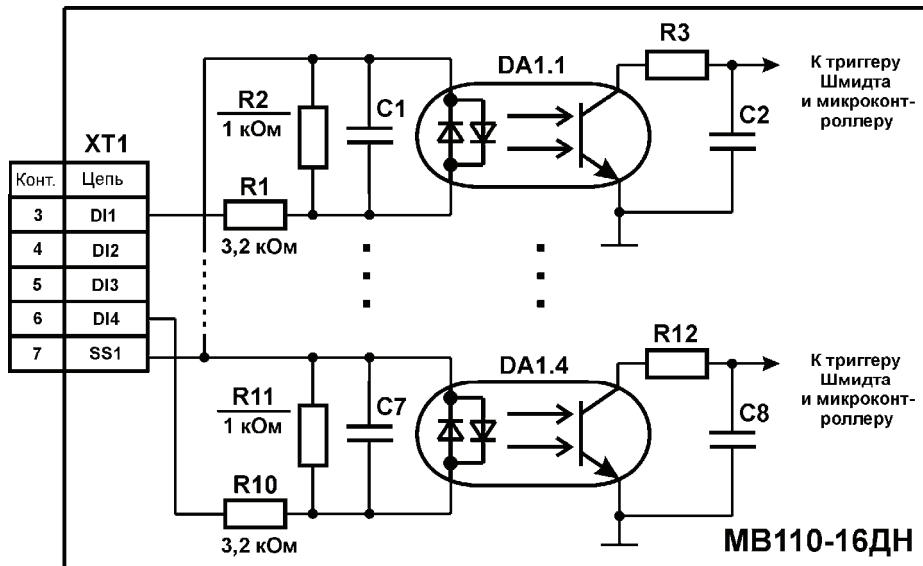
Рис. Б.8. Электрическая принципиальная схема группы дискретных входов MB110-16ДН (схема других групп входов идентична приведенной)
