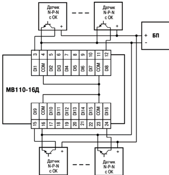
Рис. Б.3. Схема подключения к МВ110-16Д трехпроводных дискретных датчиков, имеющих выходной транзистор n-p-n- типа с открытым коллектором
