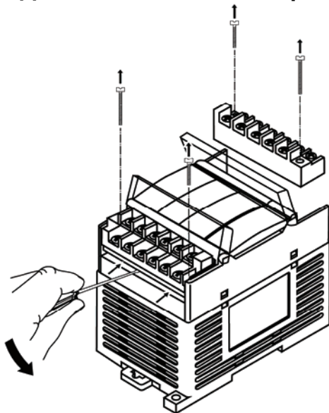
Рис. Д.1. Отделение съемных частей клемм MB110
