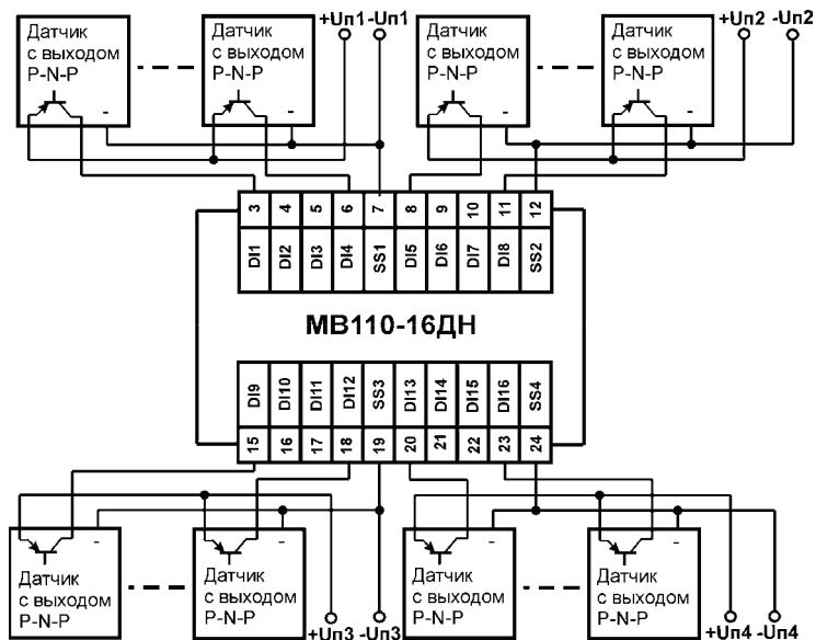
Рис. Б.6. Схема подключения к МВ110-16ДН дискретных датчиков с транзисторным выходом р-п-р-типа
