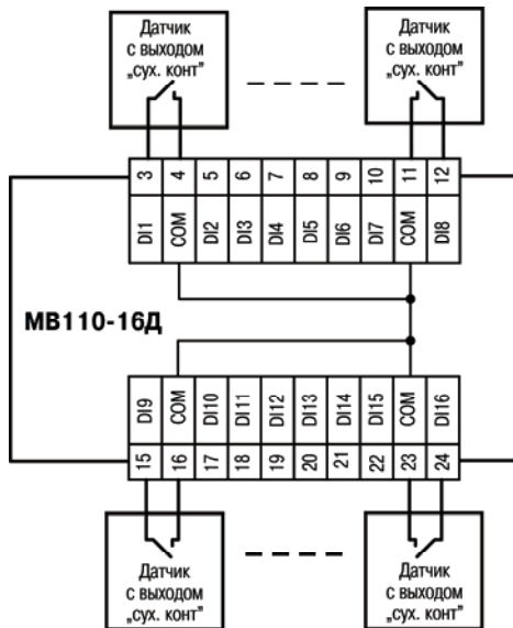
Рис. Б.2. Схема подключения к МВ110-16Д дискретных датчиков с выходом типа «сухой контакт»
