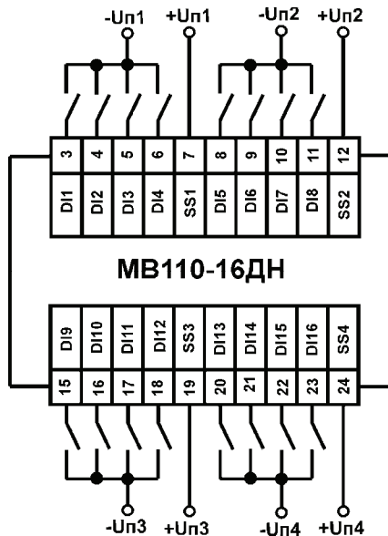
Рис. Б.4. Схема подключения к МВ110-16ДН дискретных датчиков с выходом типа «сухой контакт»
