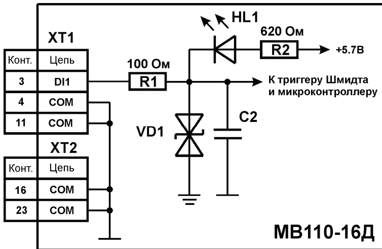
Рис. Б.7. Электрическая принципиальная схема входа MB110-16Д (схема других входов идентична приведенной)
