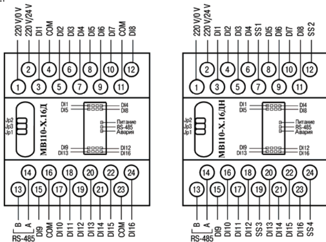
Рис. Б.1. Общий чертёж MB110
