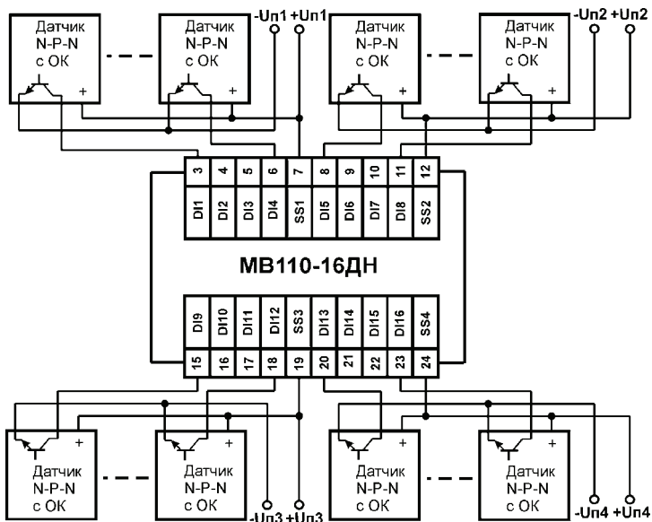
Рис. Б.5. Схема подключения к MB110-16ДН дискретных датчиков с транзисторным выходом п-р-п-типа с ОК
