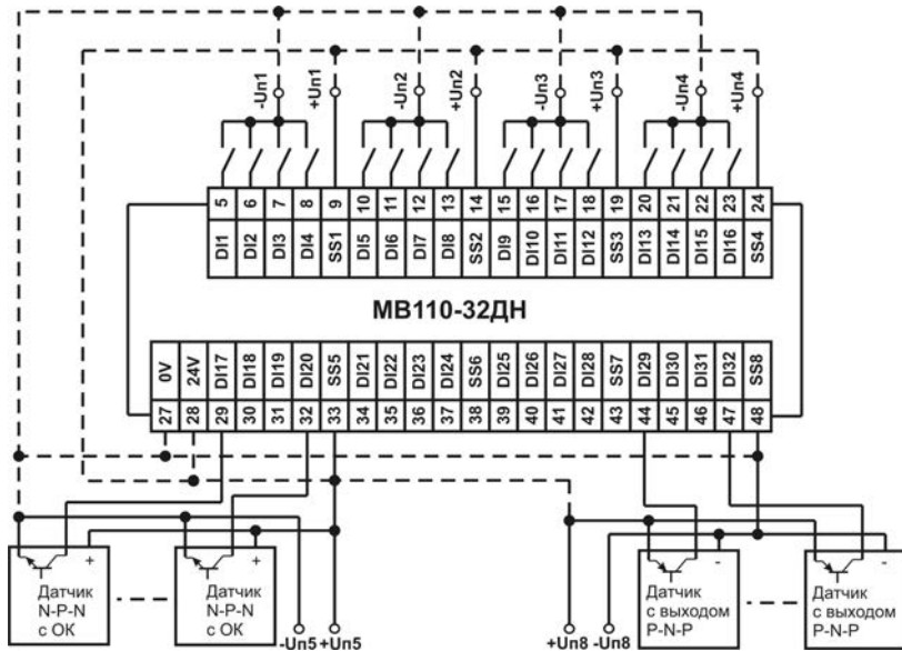
Рисунок Б.5 – Схема подключения к МВ110-32ДН дискретных датчиков с транзисторным выходом р-п-п-типа, п-р-п-типа с ОК и с выходом типа «сухой контакт» (пример)
