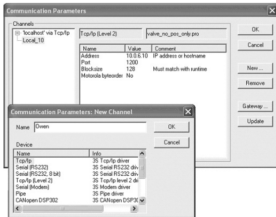
Рис. 7. Настройка коммуникационных параметров для соединения с ПЛК
