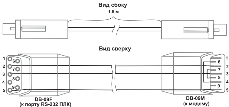
Рис. Б6. Схема кабеля подключения модема к ПЛК100 по интерфейсу V5-232
