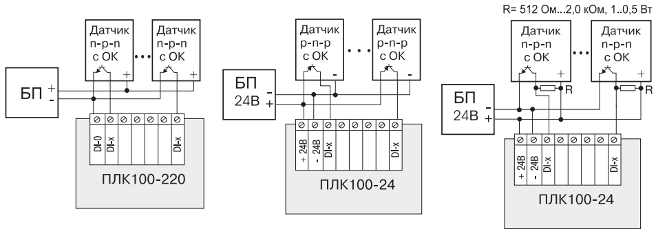
Рис. Б8. Схемы подключения к ПЛК100 дискретных датчиков с полупроводниковым выходным каскадом:
