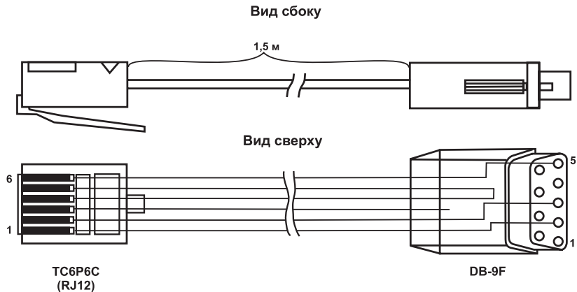
Рис. Б4. Схема кабеля программирования, входящего в комплект поставки
