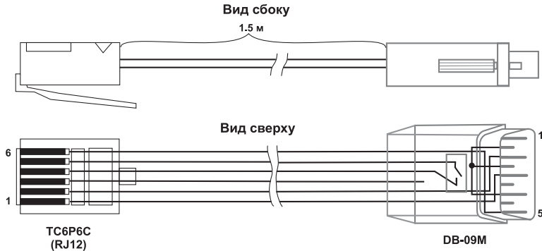
Рис. Б5. Схема "Модемный кабель ПЛК1ХХ"
