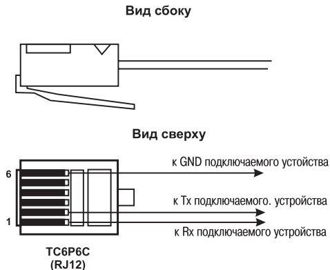
Рис. Б7. Схема кабеля для подключения к порту Debug RS-232
