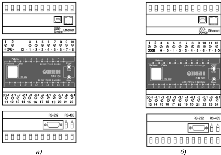
Рис. 1. Внешний вид ПЛК100-24 (а) и ПЛК100-220 (б)
