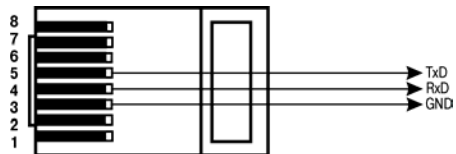
Рисунок Б.3 – Кабель связи ПЛК по RS-232 с внешним устройством
