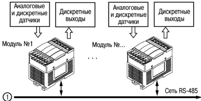
Рисунок 6.2 – Пример структуры соединений при использовании ПЛК в системе управления (продолжение)
