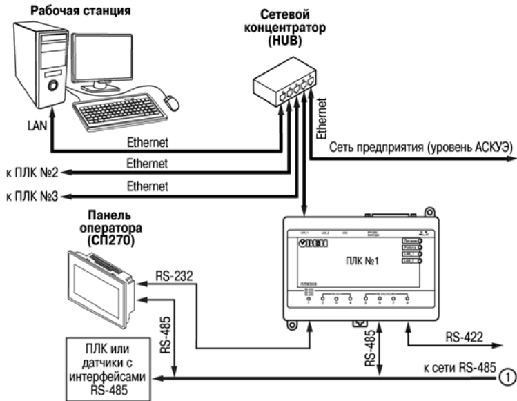
Рисунок 6.2 – Пример структуры соединений при использовании ПЛК в системе управления
