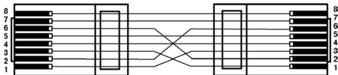
Рисунок Б.1 – Кросс-кабель для связи ПК и ПЛК через Ethernet См. также таблицу Б.1.
