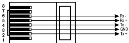
Рисунок Б.4 – Кабель связи ПЛК по RS-422 с внешним устройством
