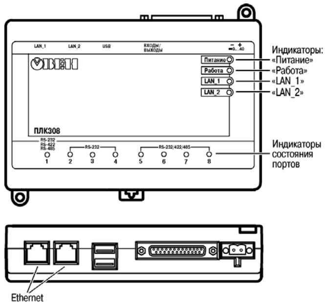
Рисунок 3.1 – Внешний вид ПЛК308
