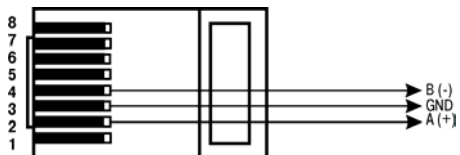
Рисунок Б.2 – Кабель связи ПЛК по RS-485 с внешним устройством
