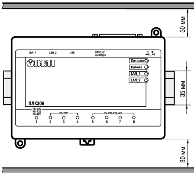
Рисунок А.3 – Расстояние до стенок корпуса ПЛК при монтаже для обеспечения вентиляции
