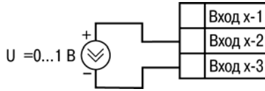
Рисунок Б.4 – Подключение активного датчика с выходом в виде напряжения 0...1 \text{ В}
