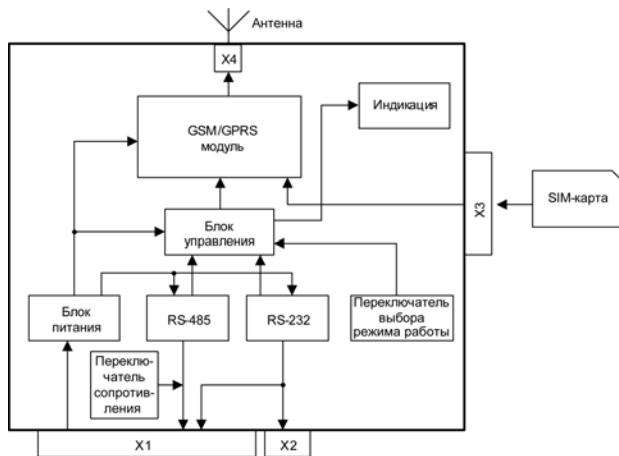
Рисунок 3.1 – Функциональная схема
