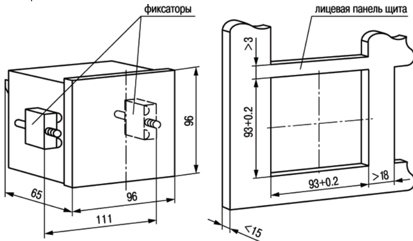
Рисунок А.3 Прибор щитового крепления Щ1
